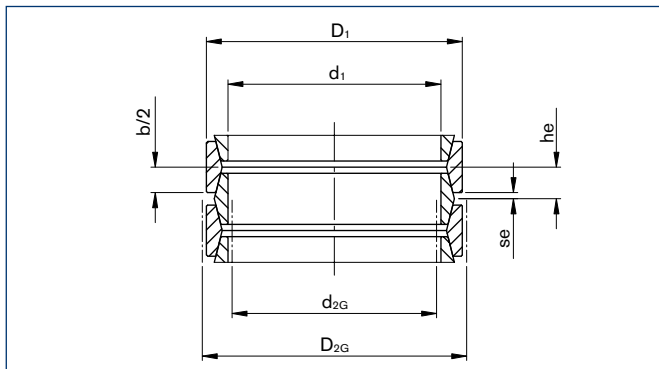
Abmessungen RINGFEDER® Reibungsfeder / Dimensions RINGFEDER® Friction Spring
