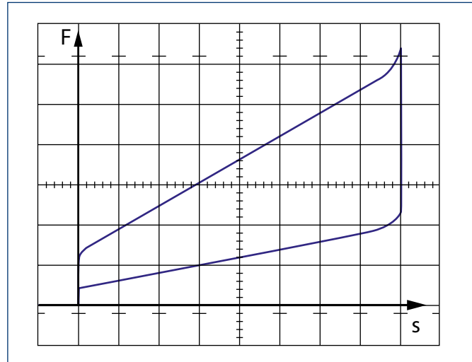
Dynamisches Kraft-Weg-Diagramm einer vorgespannten
